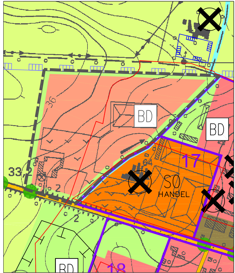
GEPLANTE DARSTELLUNG M 1:5.000 - Blatt 1 (Ausschnitt)
